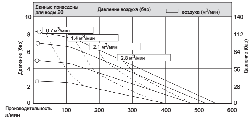
Кривые производительности
