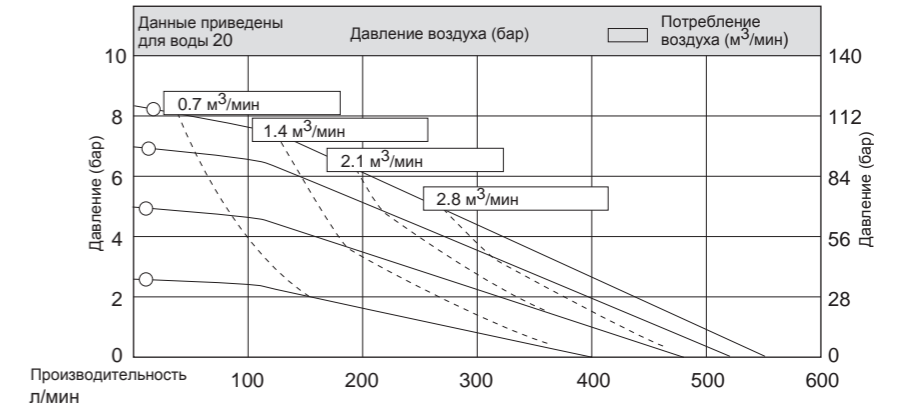
Кривые производительности
