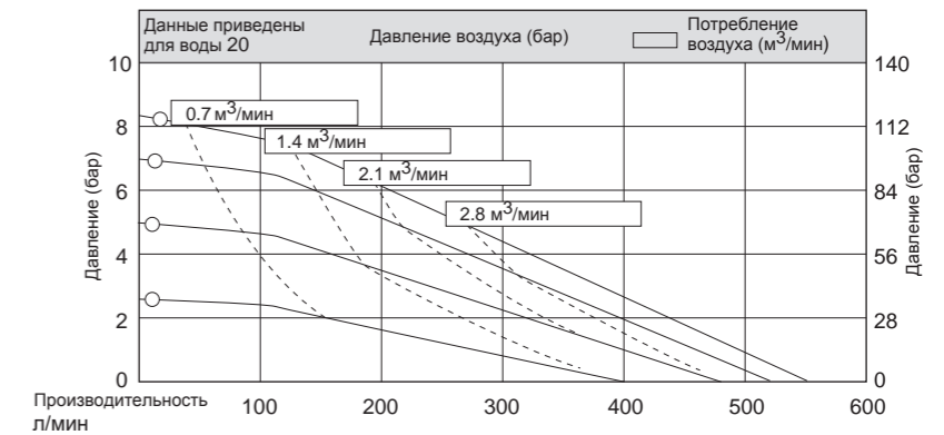
Кривые производительности
